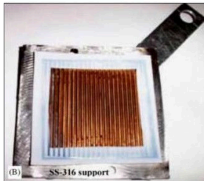
图 1-10 质子交换膜燃料电池波状铜合金双极板 [25]
