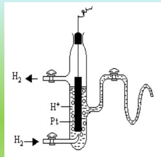
氢电极结构简图
