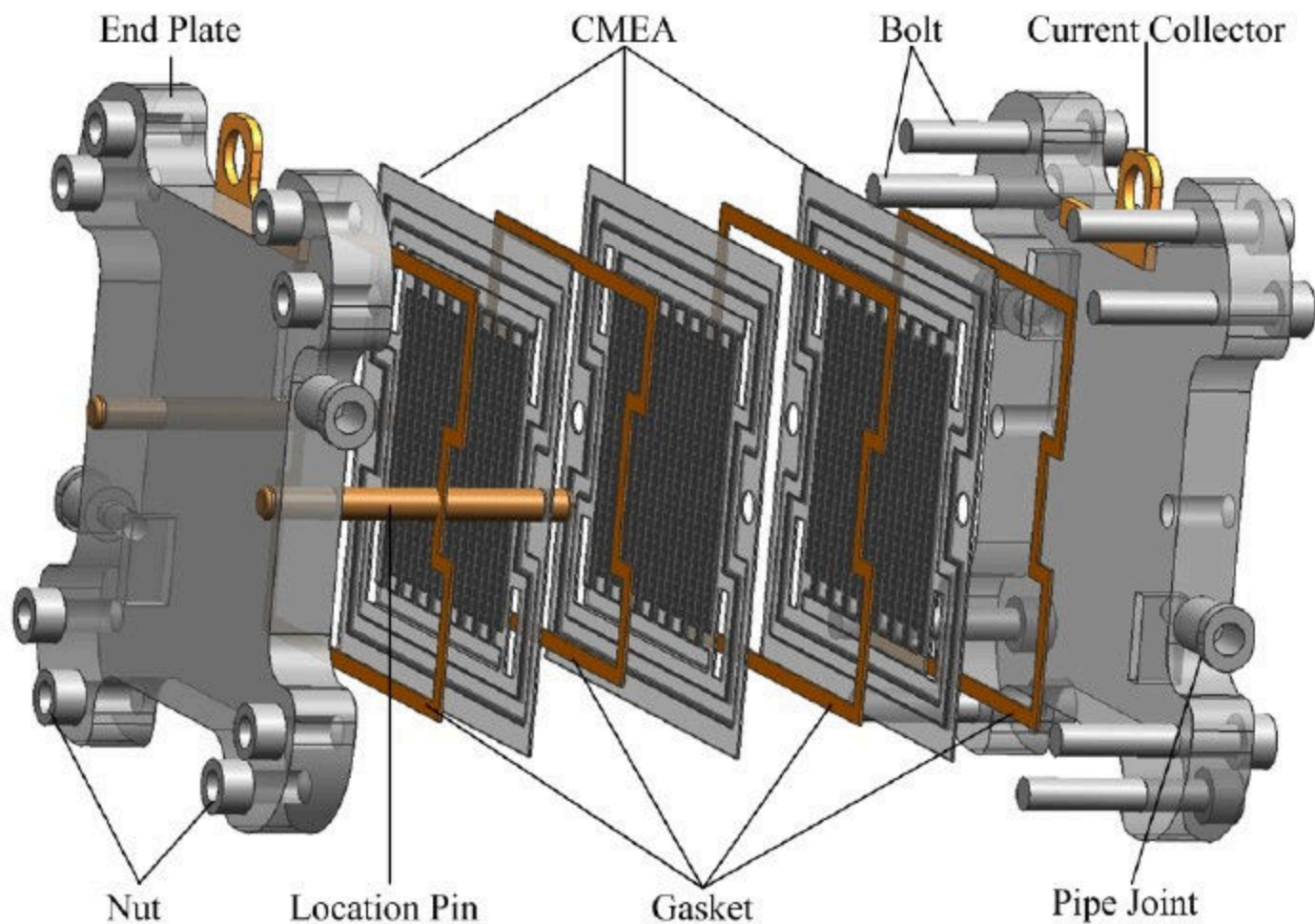
图 2-8 无极板式 PEMFC 电堆结构设计
