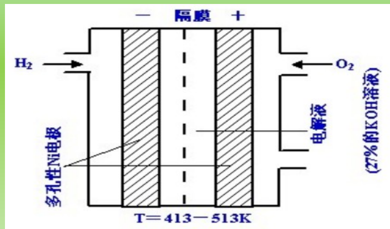
\text{H}_2 \sim \text{O}_2 燃料电池示意图
